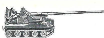
112 Feldkanone 175 mm M 107 USA, Bundeswehr M 107 Canon Automoteur de 175 mm, USA et Nato M 107 self propelled 175 cannon, USA
