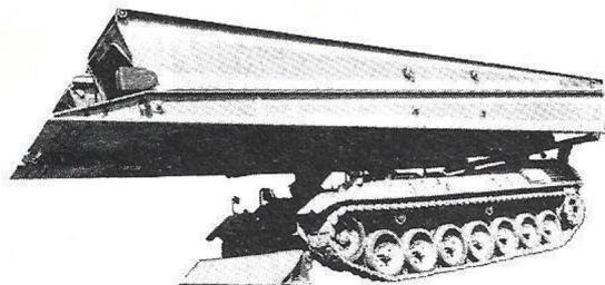
26 Brückenlegepanzer Biber mit beweglicher Brücke, Bundeswehr Char poseur, pont mobile, Allemagne Bridge layer „Beaver“ with movable bridge, Western Germany
